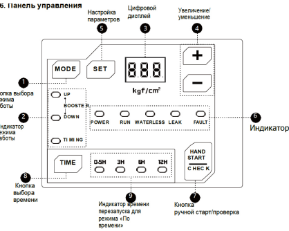
Старая версия контроллера
