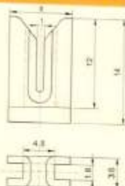
Slit Guides / 开口型导丝器
