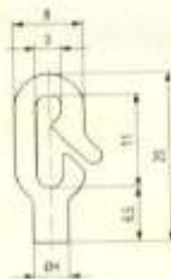
Hook Guides / 钩型导丝器
