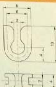
Slit Guides / 开口型导丝器
