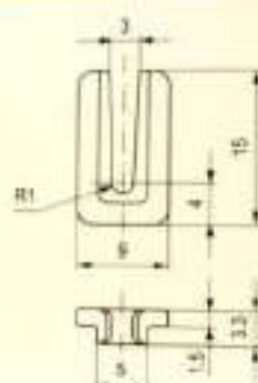
Slit Guides / 开口型导丝器
