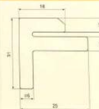
Slit Guides / 开口型导丝器
