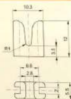
Slit Guides / 开口型导丝器
