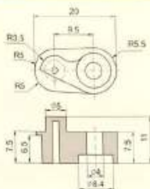
Diverse Guides / 异型导丝器
