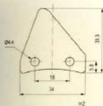
Traverse Guides / 横动导丝器
