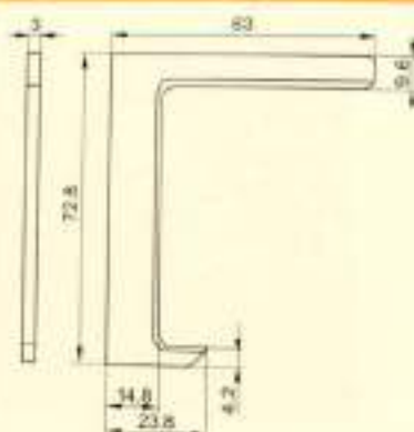
Traverse Guides / 横动导丝器
