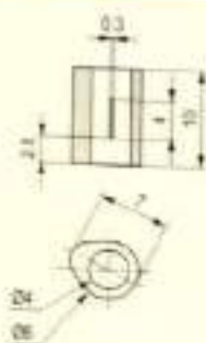
Diverse Guides / 异型导丝器
