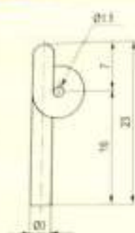
Pigtails / 猪尾型导丝器
