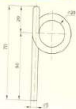
Pigtails / 猪尾型导丝器
