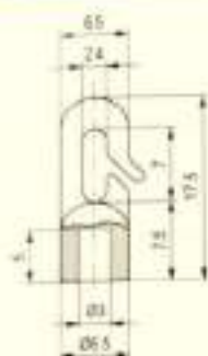
Hook Guides / 钩型导丝器
