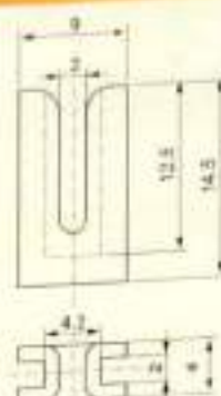
Slit Guides / 开口型导丝器
