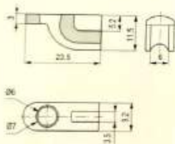
Diverse Guides / 异型导丝器
