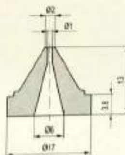
Air Jets / 气流油嘴
