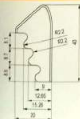
Traverse Guides / 横动导丝器
