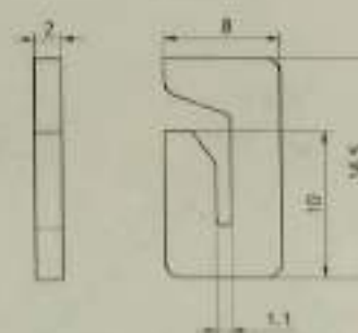
Slit Guides / 开口型导丝器
