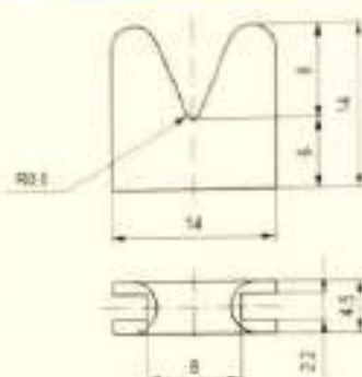
Slit Guides / 开口型导丝器
