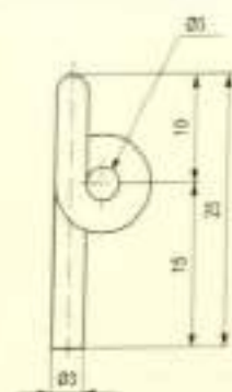
Pigtails / 猪尾型导丝器
