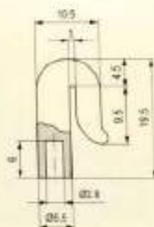
Hook Guides / 钩型导丝器
