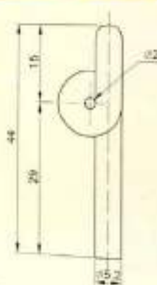
Pigtails / 猪尾型导丝器
