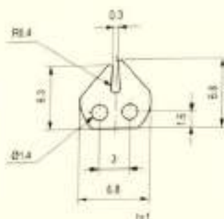
Traverse Guides / 横动导丝器
