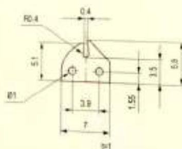
Traverse Guides / 横动导丝器
