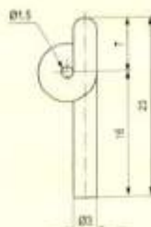
Pigtails / 猪尾型导丝器
