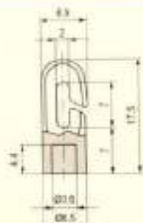
Hook Guides / 钩型导丝器
