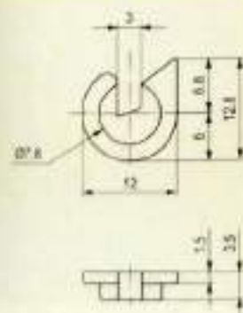
Slit Guides / 开口型导丝器
