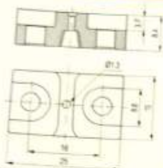
Air Jets / 气流油嘴
