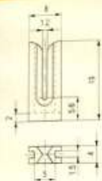
Slit Guides / 开口型导丝器
