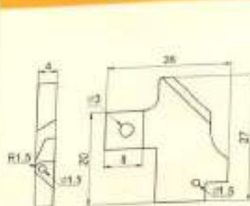
Diverse Guides / 异型导丝器
