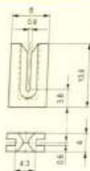
Slit Guides / 开口型导丝器
