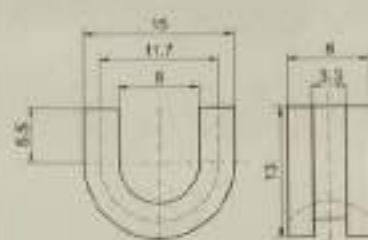
Slit Guides / 开口型导丝器
