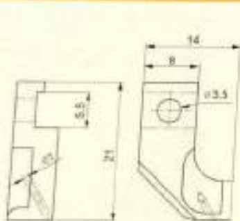
Diverse Guides / 异型导丝器
