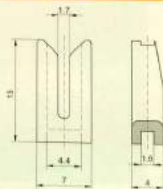
Slit Guides / 开口型导丝器
