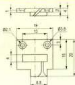
Slit Guides / 开口型导丝器
