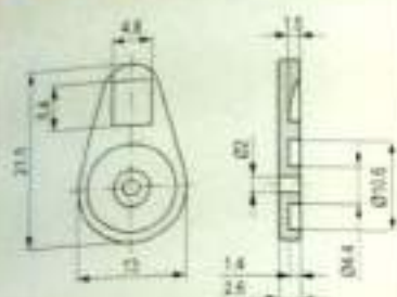
Hook Guides / 钩型导丝器
