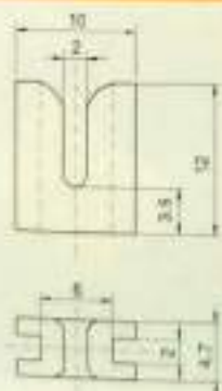
Slit Guides / 开口型导丝器
