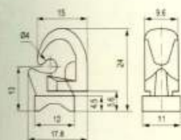
Hook Guides / 钩型导丝器
