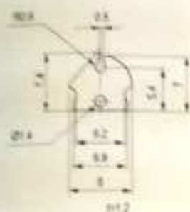
Traverse Guides / 横动导丝器
