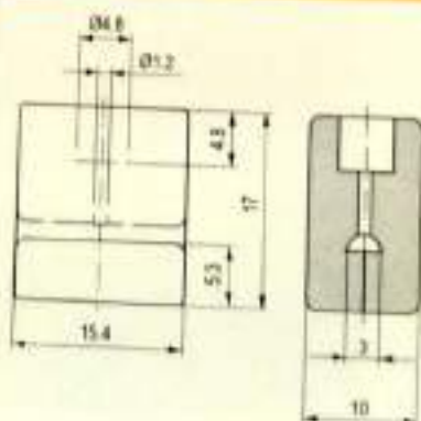
Air Jets / 气流油嘴
