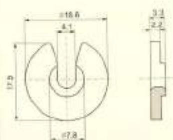
Slit Guides / 开口型导丝器
