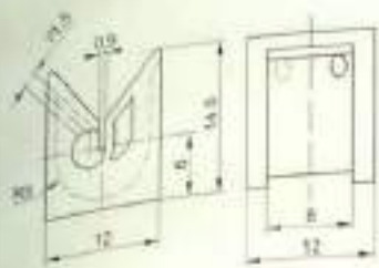
Air Jets / 气流喷嘴
