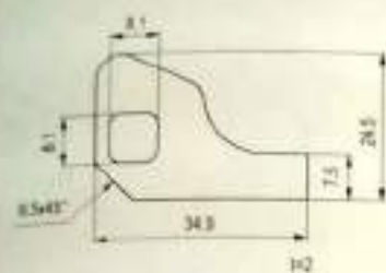
Traverse Guides / 横动导丝器
