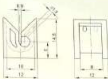
Air Jets / 气流喷嘴
