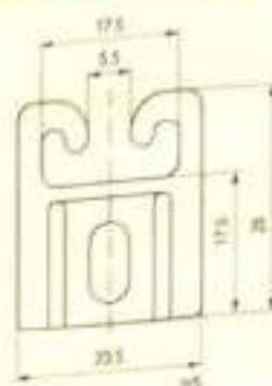
Slit Guides / 开口型导丝器
