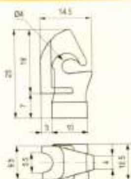
Hook Guides / 钩型导丝器
