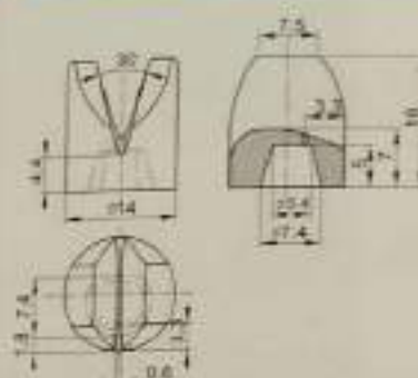
Oiling Nozzles / 上油嘴
