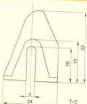
Traverse Guides / 横动导丝器
