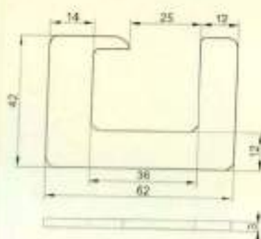
Traverse Guides / 横动导丝器
