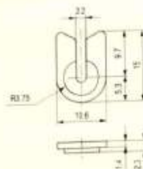
Slit Guides / 开口型导丝器
