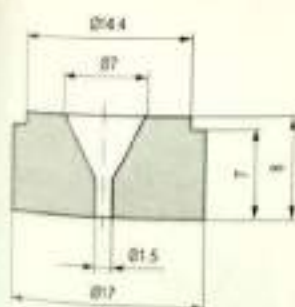
Air Jets / 气流油嘴
