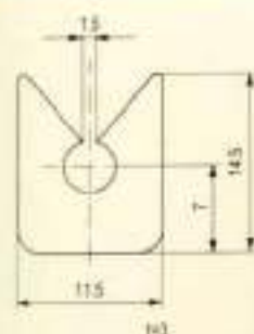
Slit Guides / 开口型导丝器
