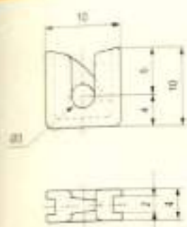
Hook Guides / 钩型导丝器
