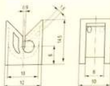
Air Jets / 气流油嘴
