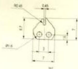
Traverse Guides / 横动导丝器
