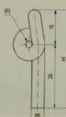
Pigtails / 猪尾型导丝器
