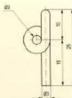
Pigtails / 猪尾型导丝器
