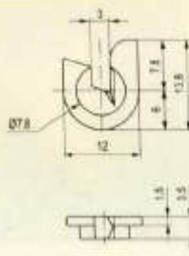
Slit Guides / 开口型导丝器
