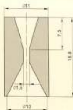
Air Jets / 气流油嘴
