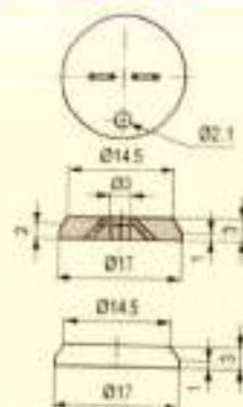
Air Jets / 气流油嘴
