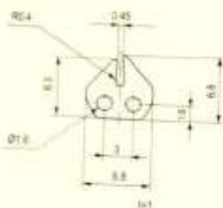
Traverse Guides / 横动导丝器
