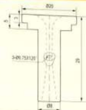
Air Jets / 气流油嘴
