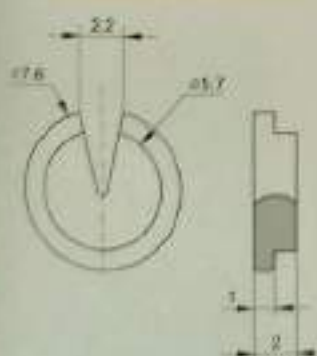
Slit Guides / 开口型导丝器
