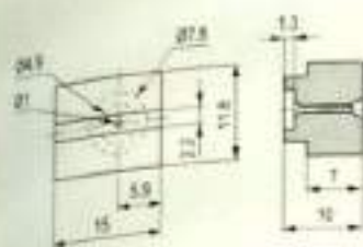
Air Jets / 气流油嘴
