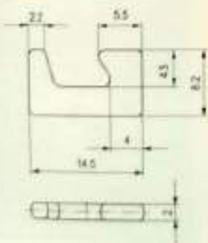
Slit Guides / 开口型导丝器
