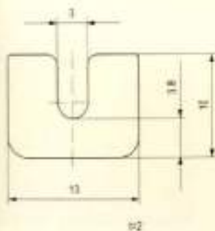
Slit Guides / 开口型导丝器
