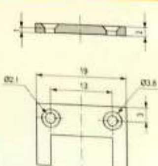
Slit Guides / 开口型导丝器
