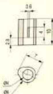
Diverse Guides / 异型导丝器
