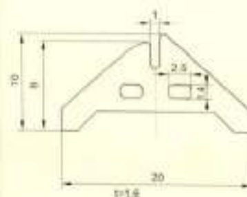
Traverse Guides / 横动导丝器
