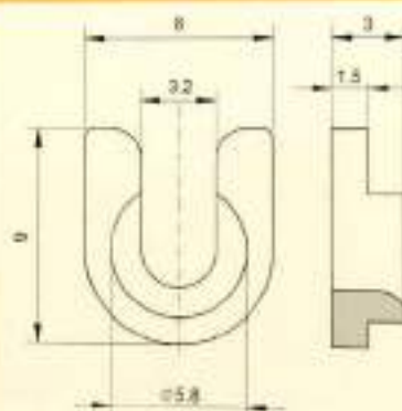
Slit Guides / 开口型导丝器
