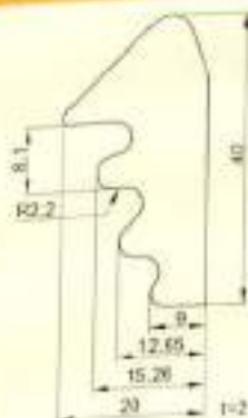
Traverse Guides / 横动导丝器
