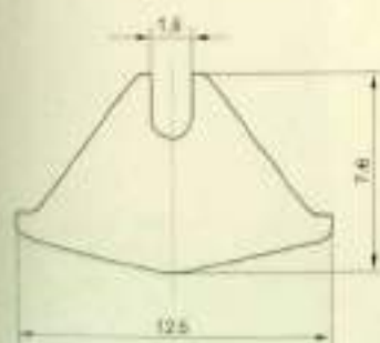
Traverse Guides / 横动导丝器
