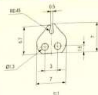
Traverse Guides / 横动导丝器
