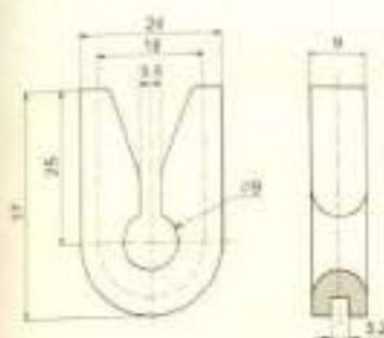
Slit Guides / 开口型导丝器
