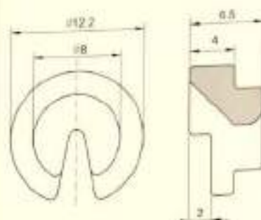
Slit Guides / 开口型导丝器
