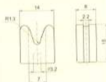
Slit Guides / 开口型导丝器
