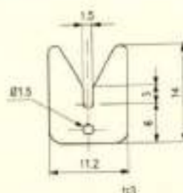
Slit Guides / 开口型导丝器
