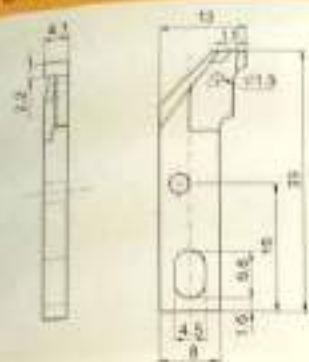
Diverse Guides / 异型导丝器
