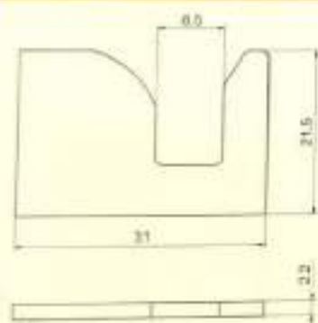
Slit Guides / 开口型导丝器
