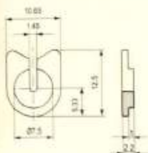
Slit Guides / 开口型导丝器
