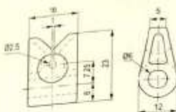
Slit Guides / 开口型导丝器
