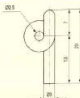
Pigtails / 猪尾型导丝器
