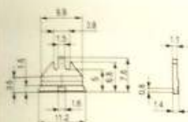
Traverse Guides / 横动导丝器
