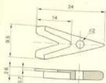
Traverse Guides / 横动导丝器
