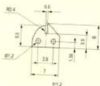
Traverse Guides / 横动导丝器
