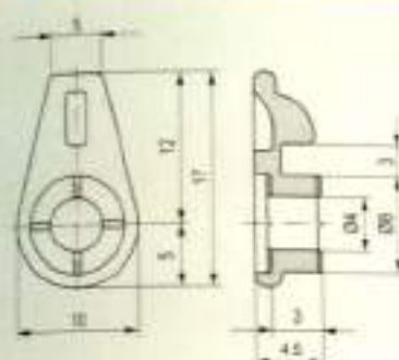
Hook Guides / 钩型导丝器
