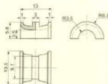
Diverse Guides / 异型导丝器
