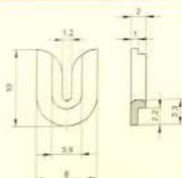
Slit Guides / 开口型导丝器
