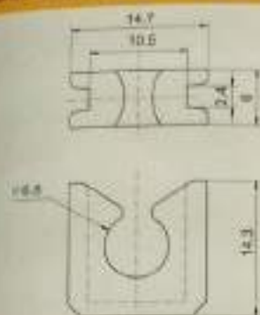
Slit Guides / 开口型导丝器
