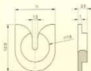
Slit Guides / 开口型导丝器
