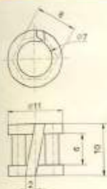
Diverse Guides / 异型导丝器
