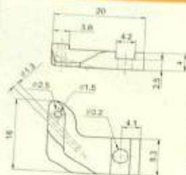
Diverse Guides / 异型导丝器
