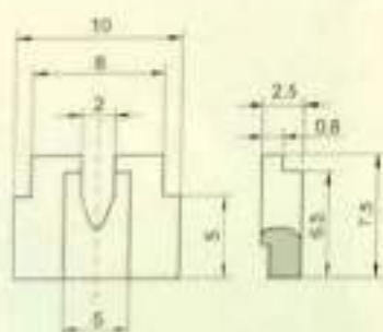
Slit Guides / 开口型导丝器
