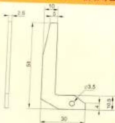
Traverse Guides / 横动导丝器
