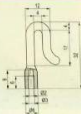
Hook Guides / 钩型导丝器
