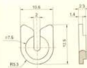
Slit Guides / 开口型导丝器
