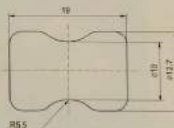
Slit Guides / 开口型导丝器
