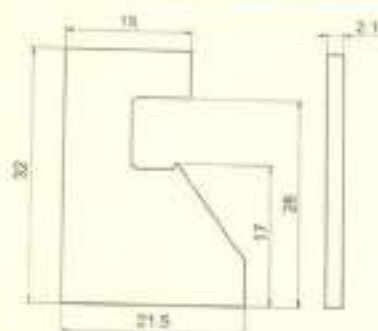
Slit Guides / 开口型导丝器
