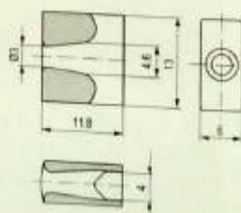
Diverse Guides / 异型导丝器
