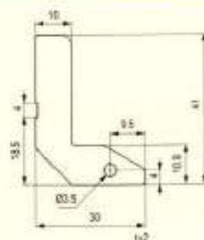
Traverse Guides / 横动导丝器
