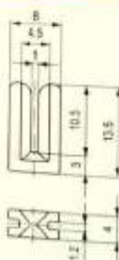
Slit Guides / 开口型导丝器
