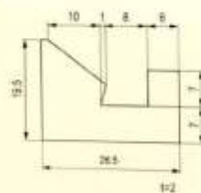
Slit Guides / 开口型导丝器
