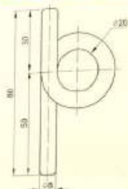
Pigtails / 猪尾型导丝器
