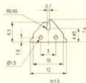
Traverse Guides / 横动导丝器
