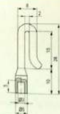
Hook Guides / 钩型导丝器
