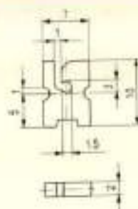
Slit Guides / 开口型导丝器
