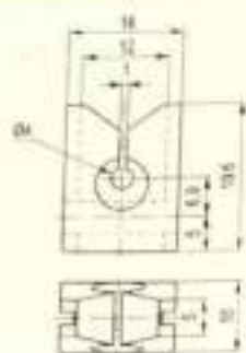
Slit Guides / 开口型导丝器
