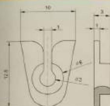
Slit Guides / 开口型导丝器
