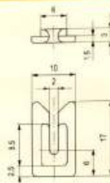
Slit Guides / 开口型导丝器
