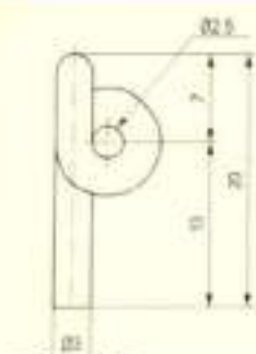
Pigtails / 猪尾型导丝器
