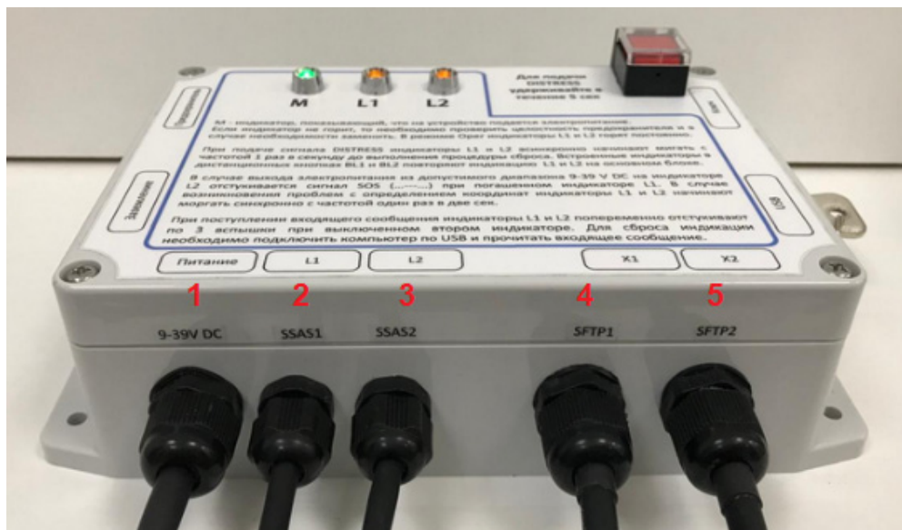
Рис.7 Назначение гермовводов на БУД
