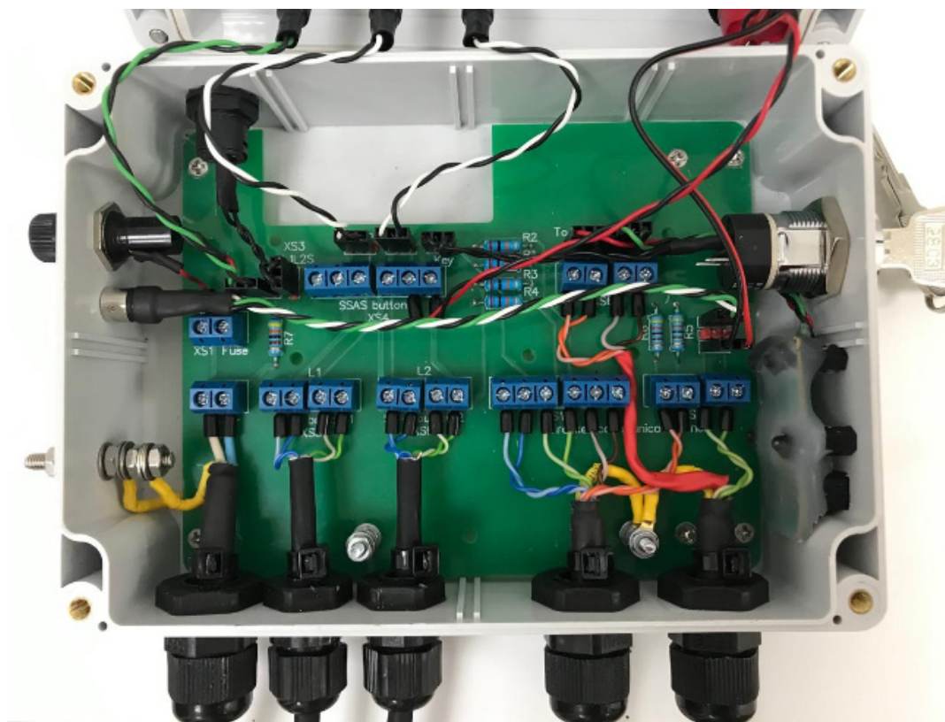
Рис.9 Образец подключения проводов на плате БУД
