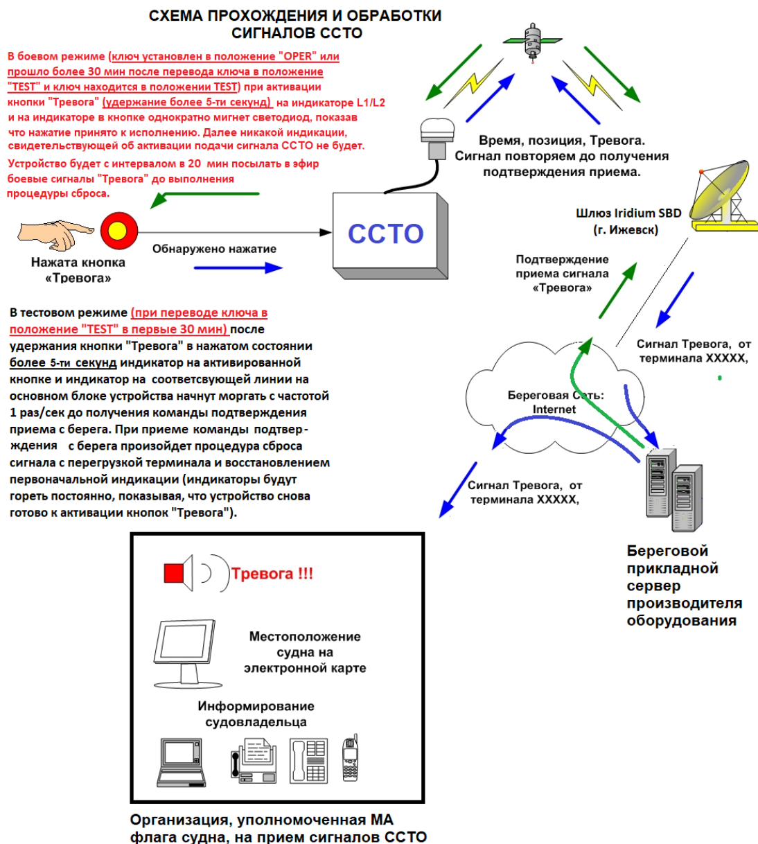
Рис. 12 Схема прохождения и обработки сигнала ССТО
