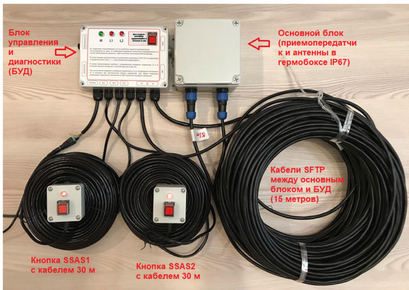
Рис. 2 Внешний вид изделия
