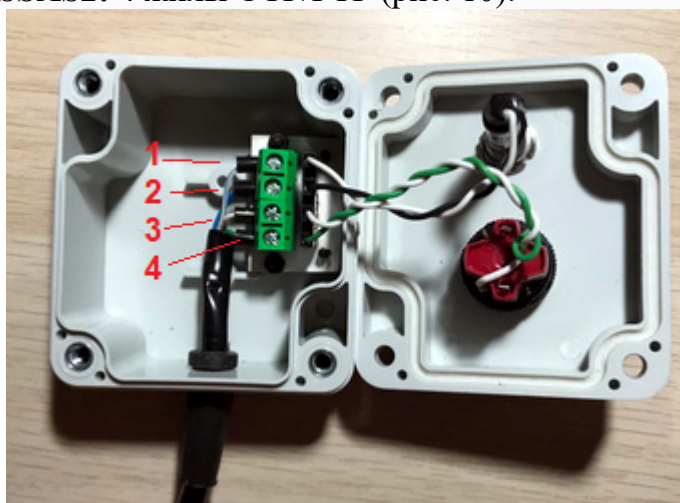
Рис. 10 Рекомендуемая расцветка жил кабеля UTP/FTP/SFTP для подключения кнопок SSAS1 и SSAS2
