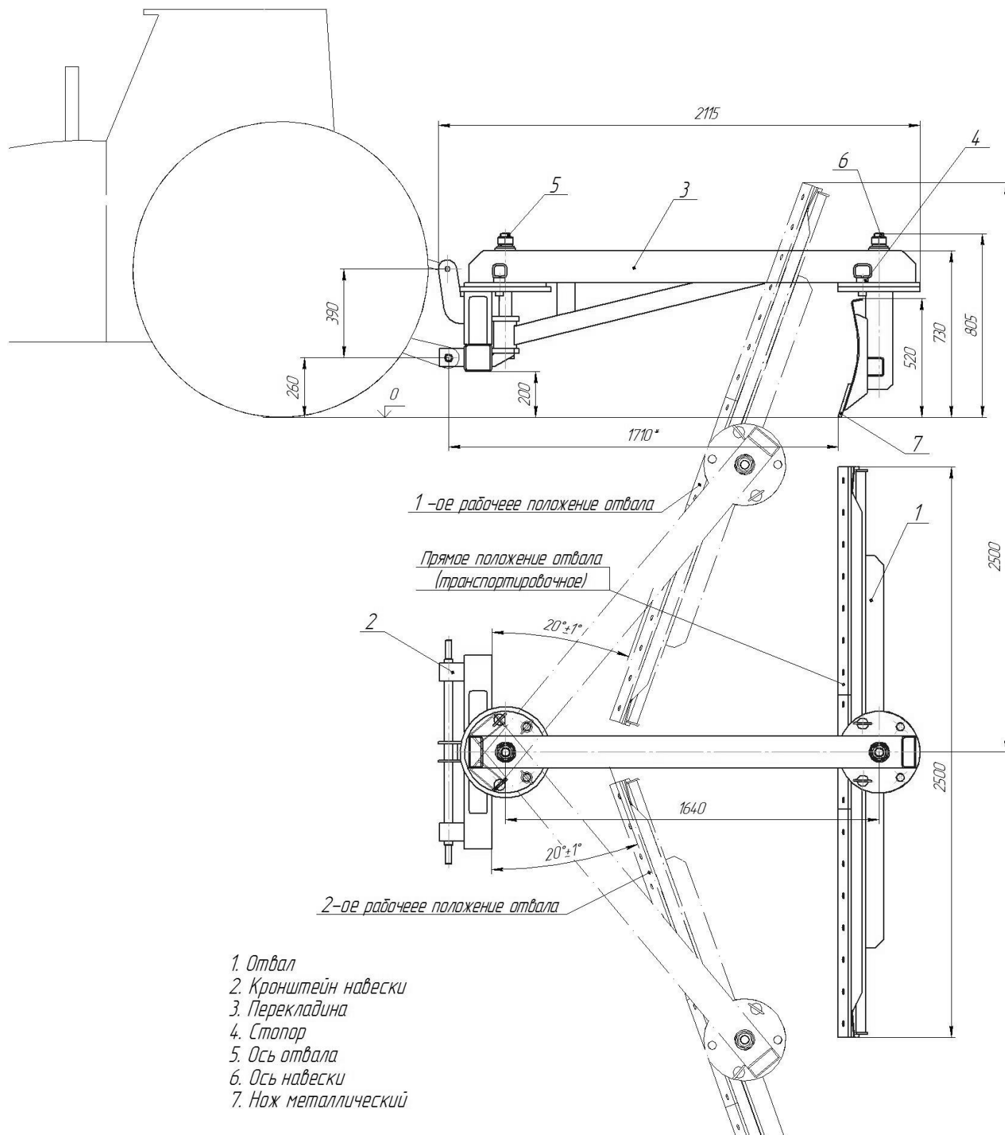
Рис.1 Отвал грейдерный на задней навеске ОБ-26
