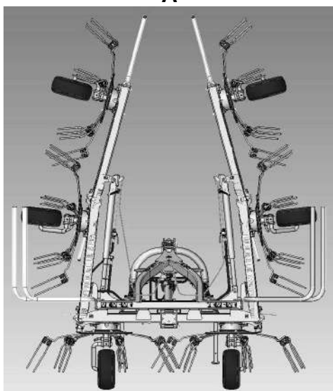
РИСУНОК 4.2А Положения ворошилки-вспушивателя
