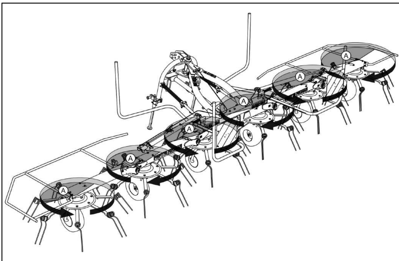
РИСУНОК 3.3А Принцип действия ворошилки-вспушивателя
