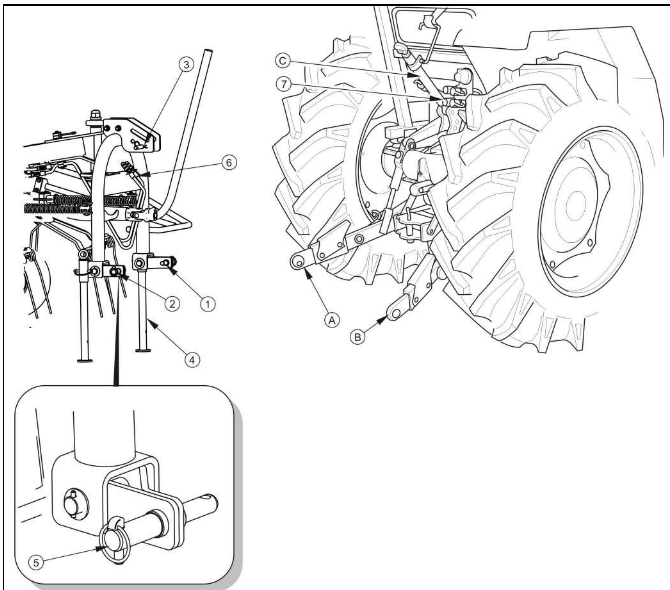
РИСУНОК 4.1А Подсоединение ворошилки-вспушивателя к трактору
