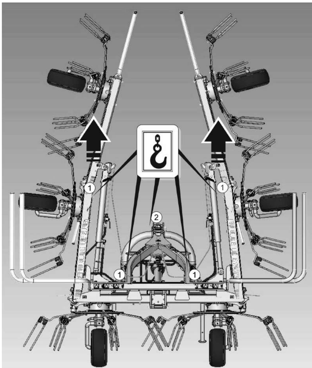
РИСУНОК 1.2А Места крепления ворошилки-вспушителя при подъеме
