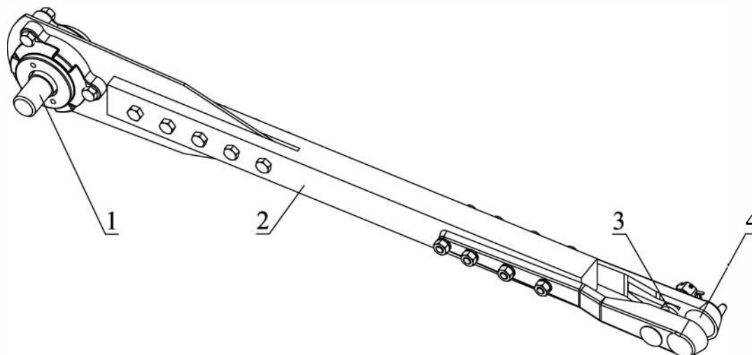
Рис. 4. Шатун.
