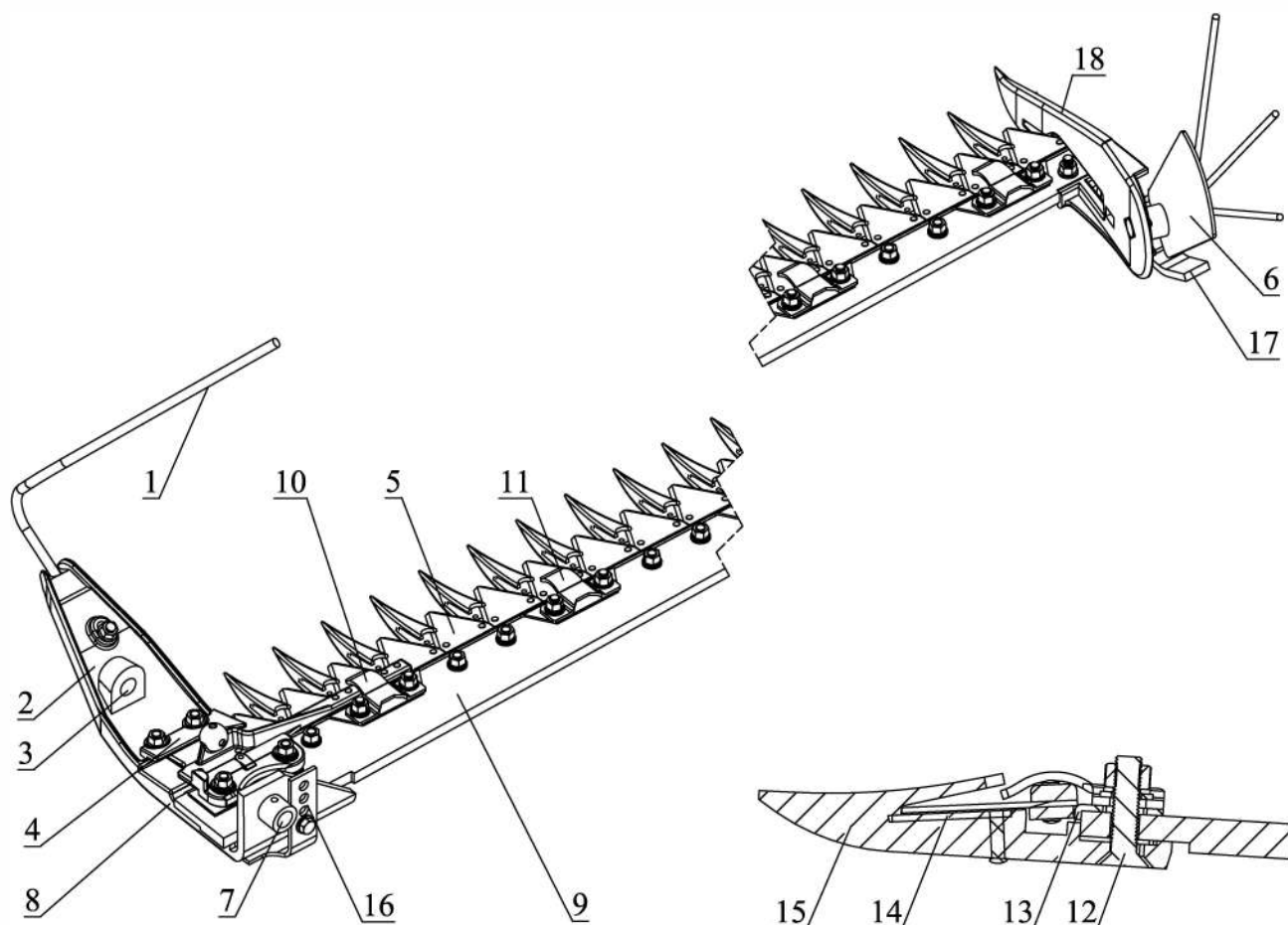
Рис. 3. Режущий аппарат.
