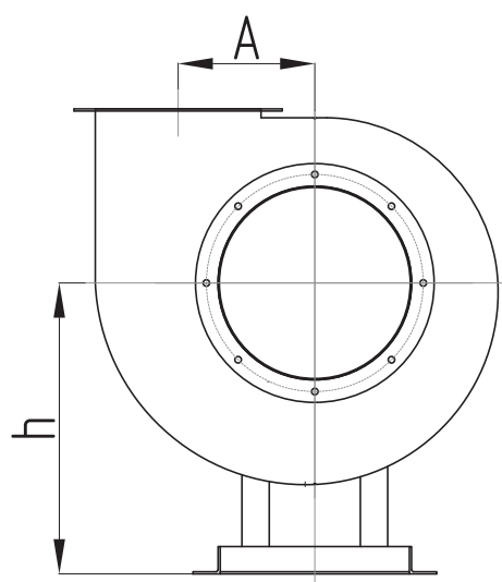
Выходной фланец
