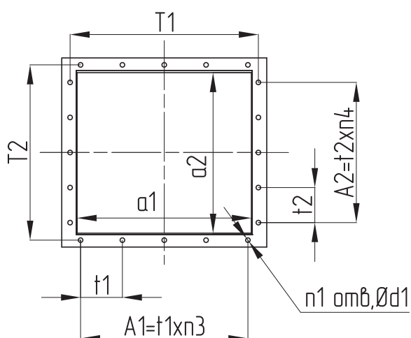
Выходной фланец
